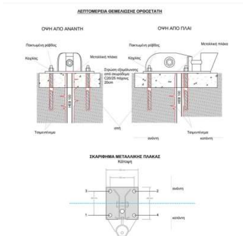
Εικόνα 6: Περιοχή IV - Λεπτομέρεια θεμελίωσης
